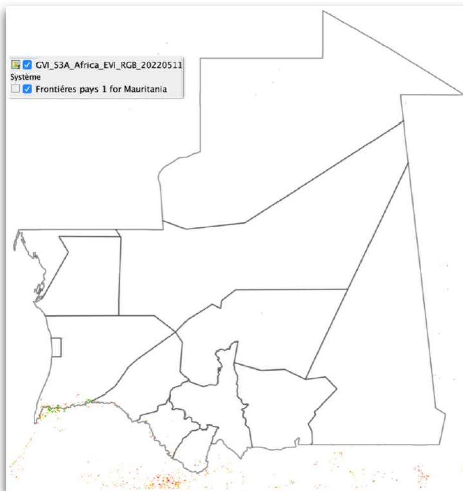
FIGURE 3 : CARTES DE VERDISSEMENT DU 11/05/2022 APPARITION DU COUVERT VEGETAL ANNUEL ENCORE TRES LOCALISES DANS LA BANDE SUDE DU PAYS
