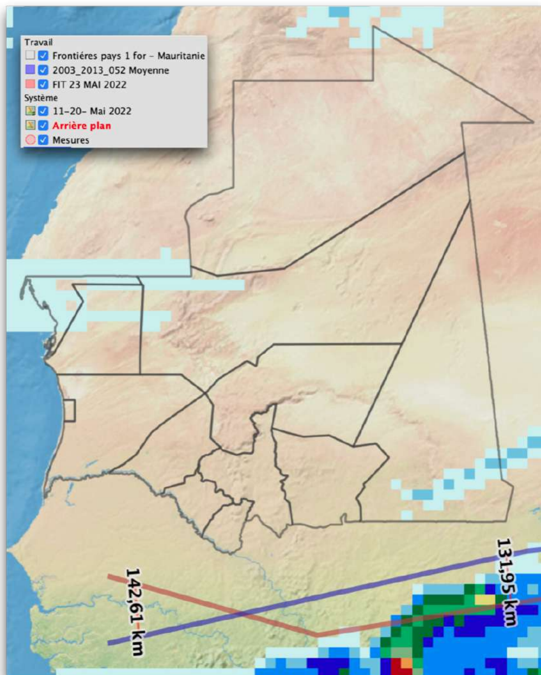
FIGURE 2 : CARTES DE PLUVIOMETRIQUES DE LA DECADE DU 11 AU 20 MAI 2022 (IRI-COLUMBIA)
