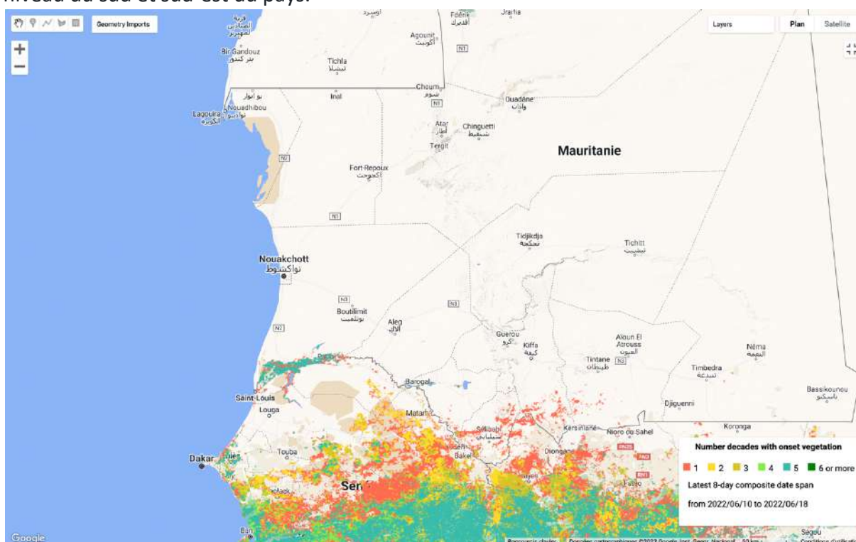
FIGURE 3 : CARTES DE VERDISSEMENT DU 10 AU 18/06/2022 APPARITION DU COUVERT VEGETAL ANNUEL AU NIVEAU DU SUD DE GUIDIMAGA, ASSABA ET HODH ECHARGUI (SOURCE GOOGLE ENGINE)
