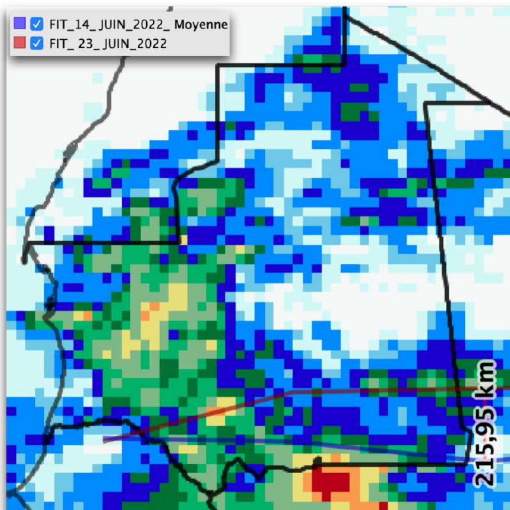
FIGURE 2 : CARTES DE PLUVIOMETRIQUES DE LA DECADE DU 11 AU 20 JUIN 2022 (IRI-COLUMBIA)
