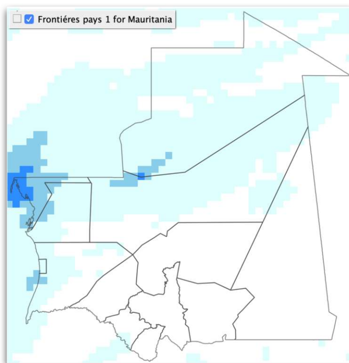
FIGURE 1 : CARTES DE PLUVIOMETRIQUES NOVEMBRE 2021 (IRI-COLUMBIA) LEGERES PRECIPITATIONS ENREGISTREES AU COURS DE CETTE PERIODE
