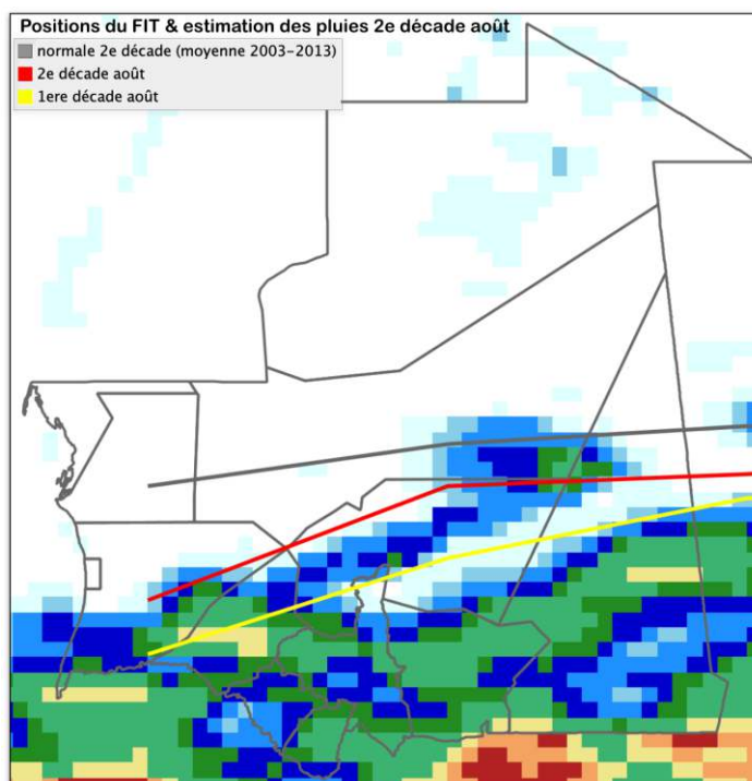
FIGURE 1 : CARTE DE PLUIES 2EME DECADE (IRI) AVEC LA SITUATION DU FIT
