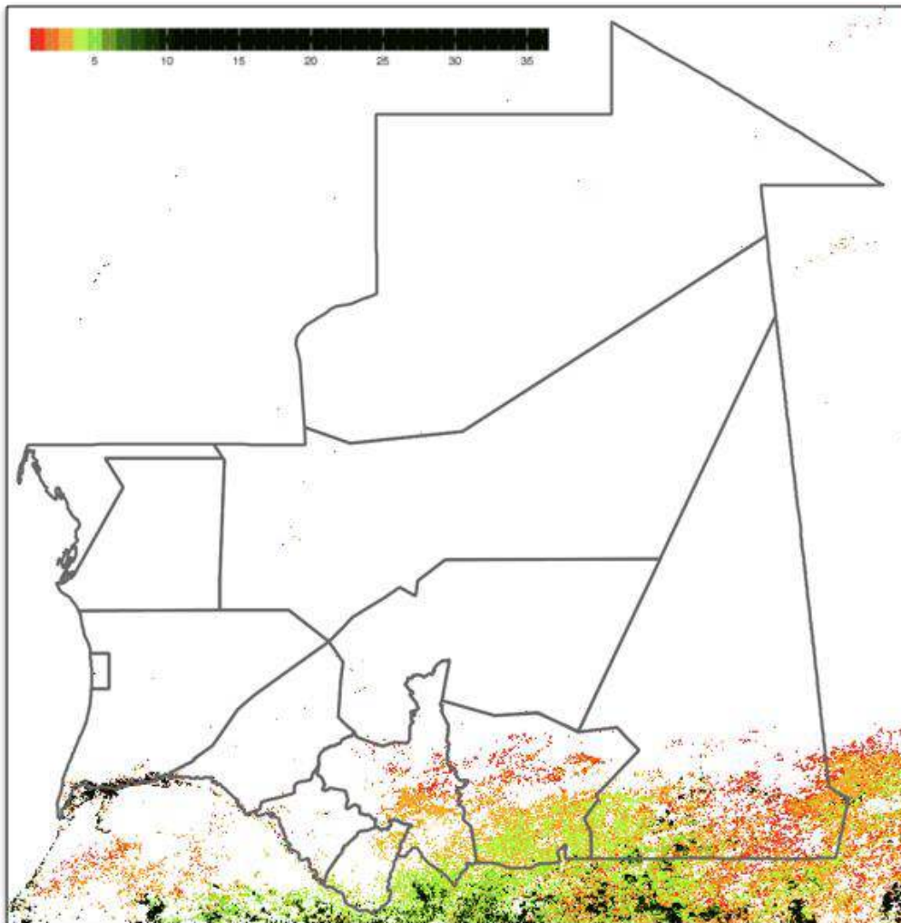
FIGURE 2 : CARTE DE SITUATION DE LA COUVERTURE VEGETALE UN REVERDISSEMENT AVANCE OBSERVE SUR LA BANDE SUDE DU PAYS (IMAGE G.A.)
