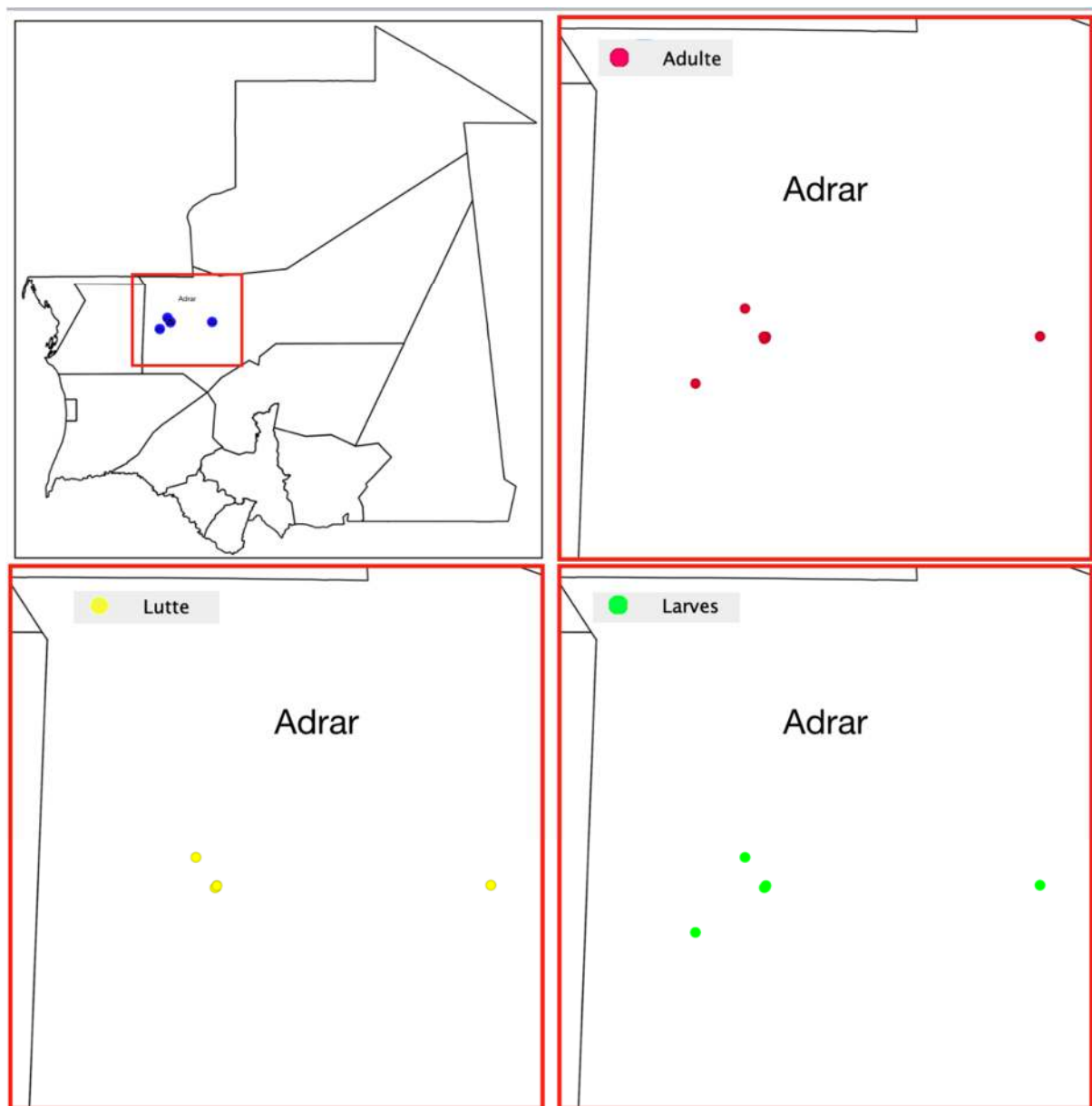
FIGURE 1 : CARTE DE SITUATION ACRIDIENNE (AVRIL 2019) Présence de larves et d'ailés au niveau de la Gara de Yaghref en Adrar
